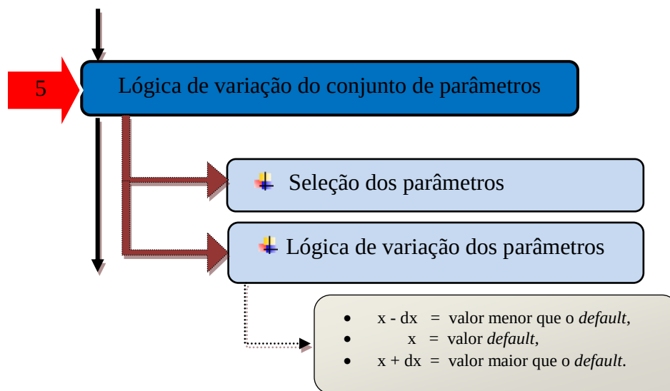
Figura 4-6: Etapa 05 do fluxograma do procedimento proposto
