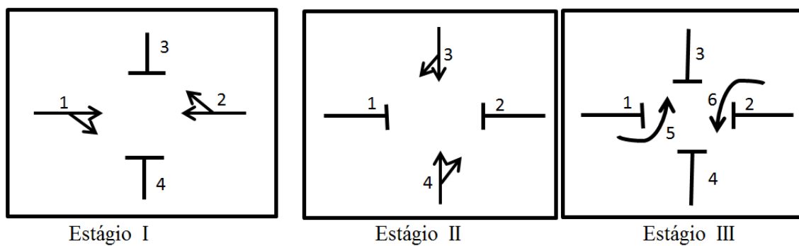
Figura A-2: Diagrama de estágios para cálculo de tempos semaforicos no projeto
