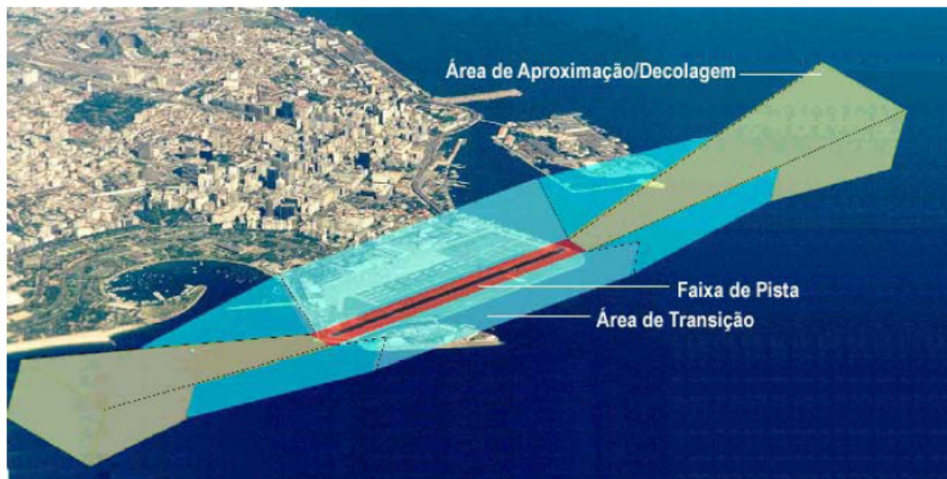
Figura 4 - Plano de Zona de Proteção de Aeródromo
